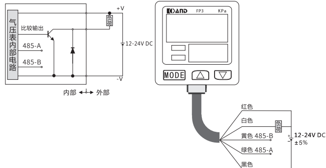
■ I/O电路图
